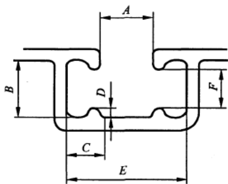
图 C.2 浇注型材槽口示意图
