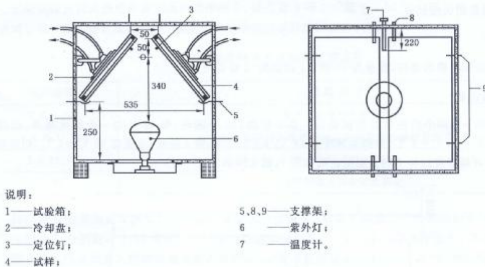
图5 紫外线试验箱
