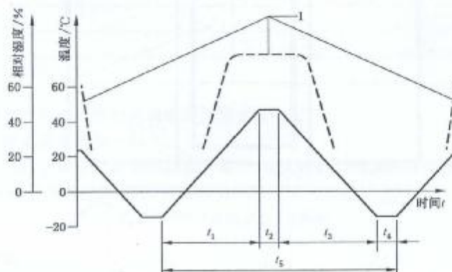
图 7 水气密封耐久性试验温度曲线
